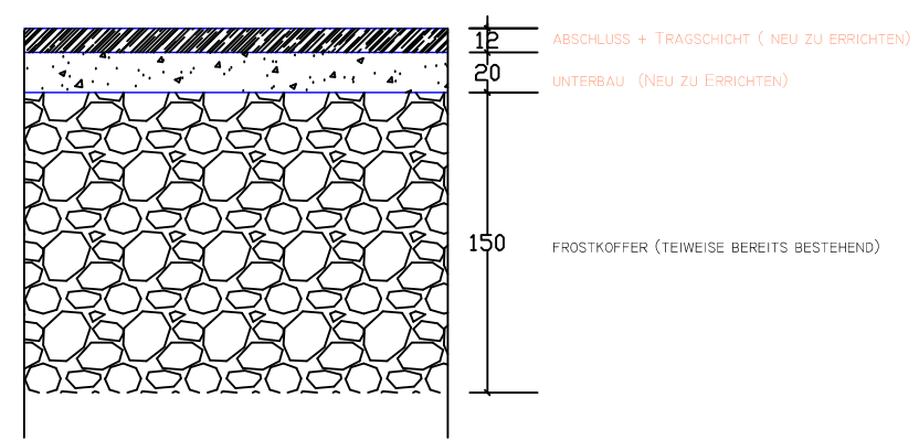
DETAIL PARKPLATZAUFBAU 1:25
